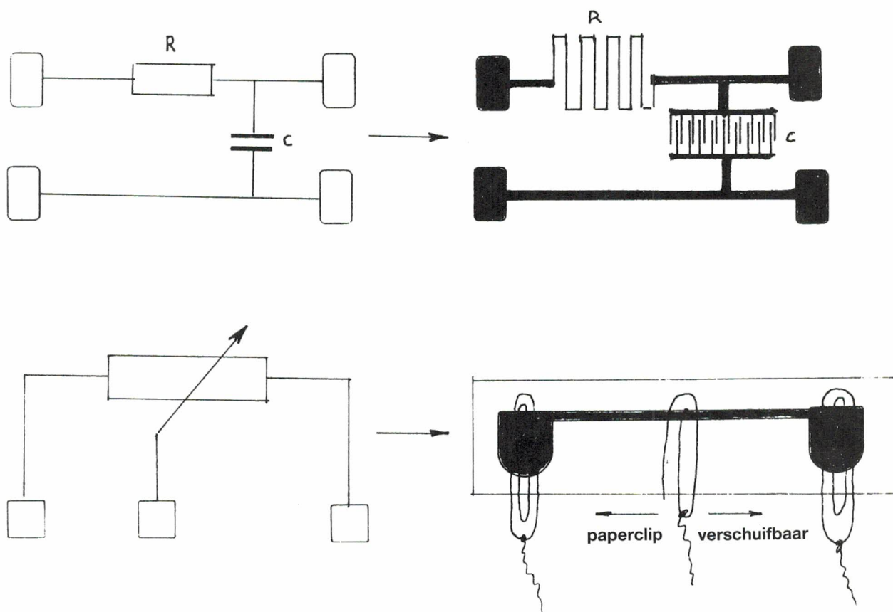
Fig. 1. Lowpassfilter en potmeter in printtechniek.
