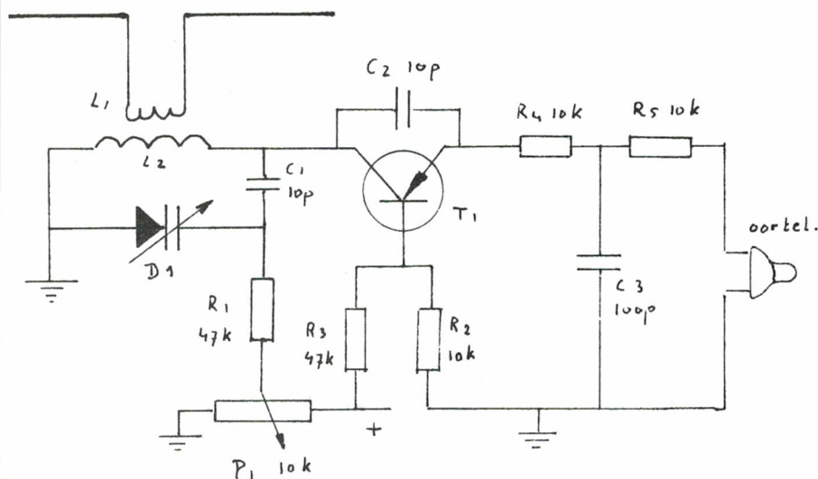
Fig. 2. Principeschema super-reg ontvanger 60-90 MHz voor kopieerprint.
