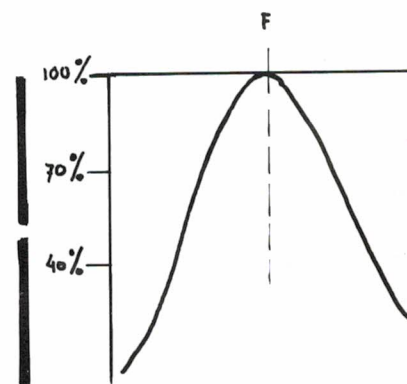
Fig. 2. Ontvangstprestaties van een dipool.
