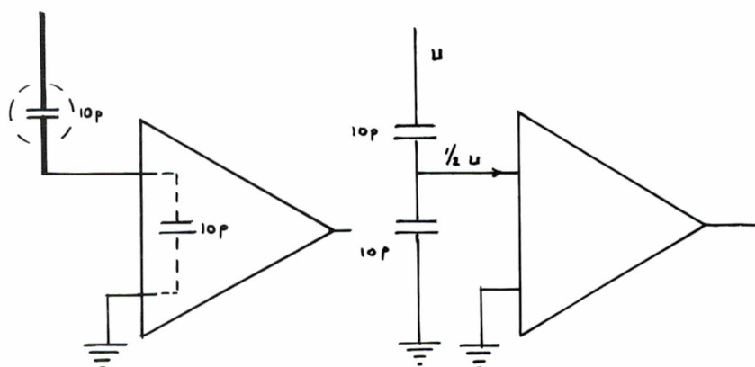
Fig. 1. Een antennespriet heeft een inwendige impedantie van ca. 10 pf. De ingangscapaciteit van de versterker zorgt voor een aanzienlijk verlies.
