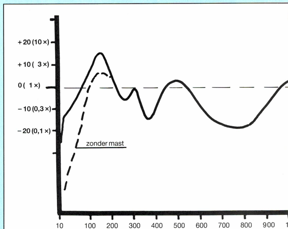
Fig. 5. Overdrachtskarakteristiek Skipmaster ASA 5050 antenne.
